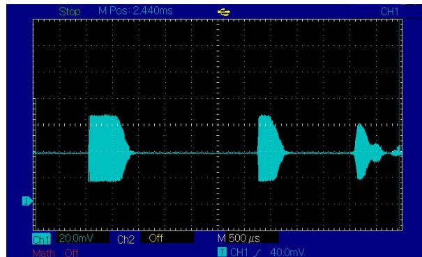
图 3：声压灵敏度
